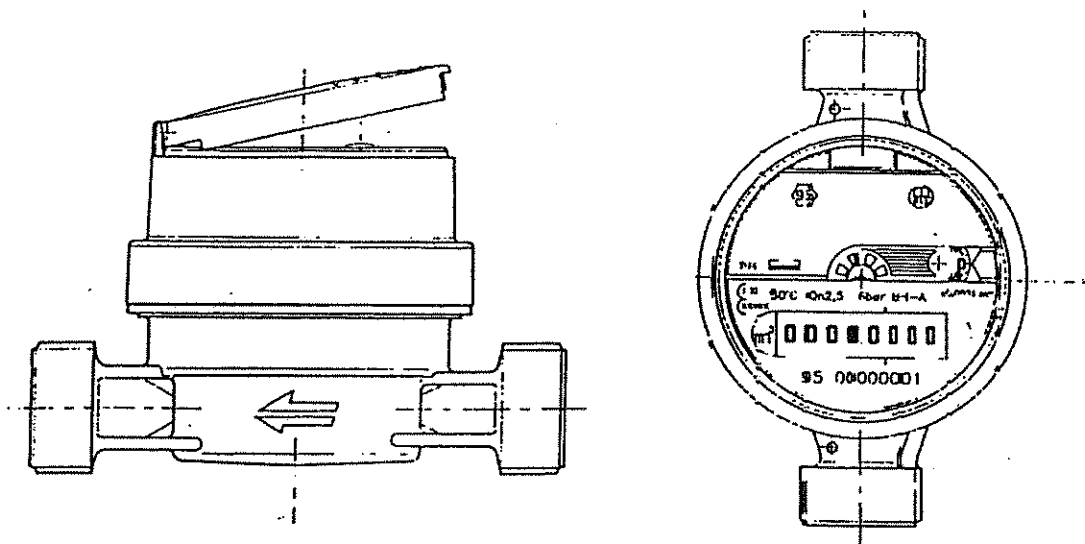
Obr. č. 7 Vodomer typu SU 4 - Unimag
