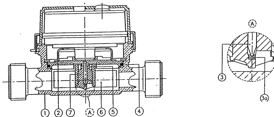
Obr. č. 3 Rez vodomerom
