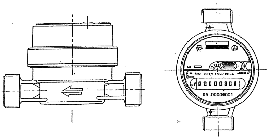
Obr. č. 8 Vodomer typu SU 4 - Marathon
