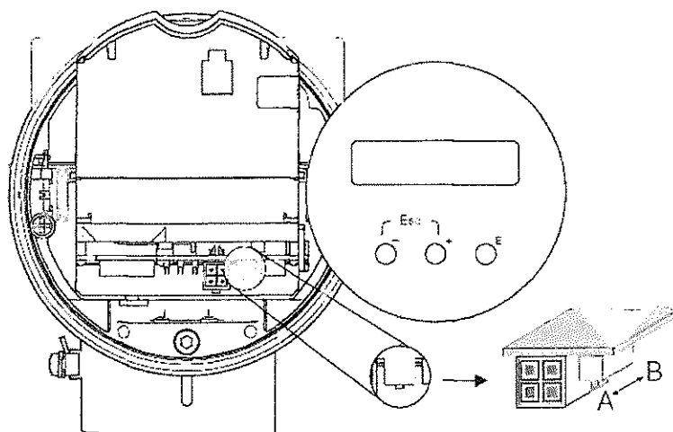
A = ochrana zápisu neaktívna (DIP-prepínač vpredu) B = ochrana zápisu aktívna (DIP-prepínač vzadu)
