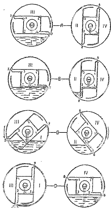
Obr.č.:3 Schéma činnosti komorového bubna
