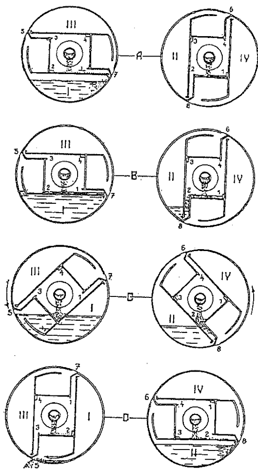
Obr.č.:2 Schéma činnosti komorového bubna
