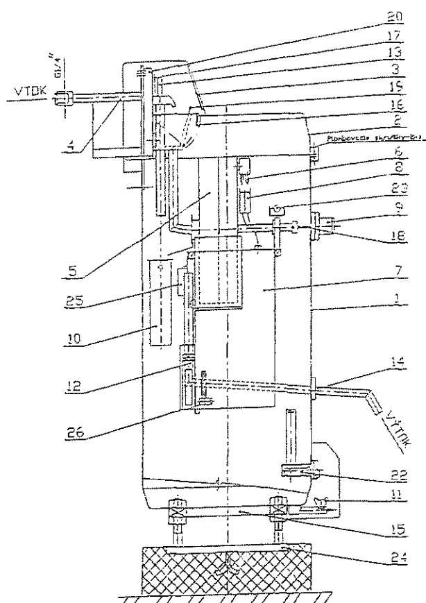
Obr.č.:1 Hlavná zostava kontrolného objemového meradla
