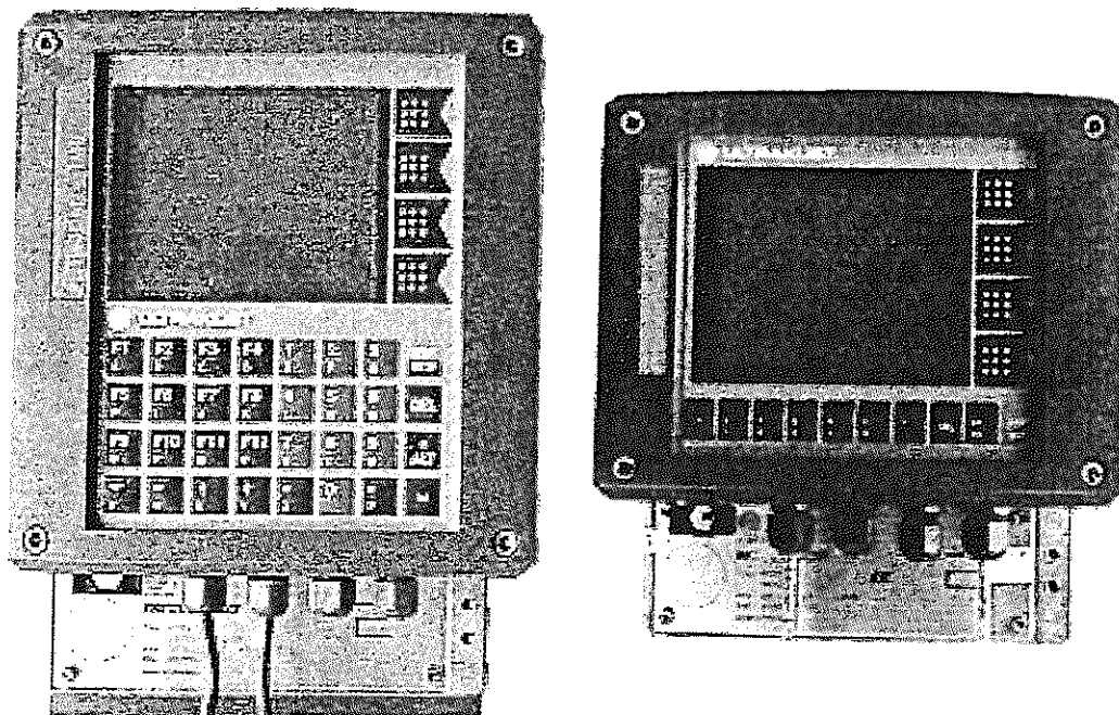
Obr.5b Centrálna riadiaca jednotka Systém (PETRODAT) 3003 Zobrazovacia a obslužná jednotka 6922-11 (Metrologické dáta/-prepínač proti zmenám)
