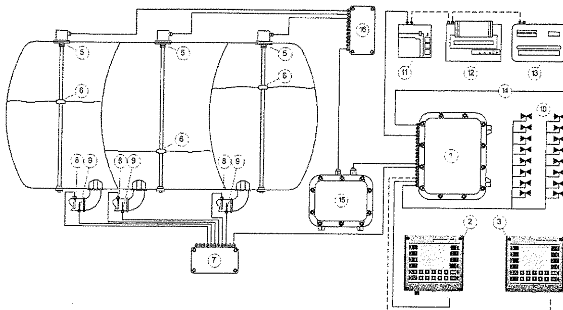
Obr. 4d Merací systém s prepočítavačom System (PETRODAT) 3003 so zásuvným rozhraním hladinomerov a snímačom náklonu (varianta 1)
