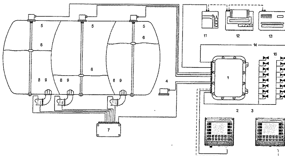
Obr. 4e Merací systém s prepočítavačom System (PETRODAT) 3003 so zásuvným rozhraním hladinomerov a snímačom náklonu (varianta 2)
