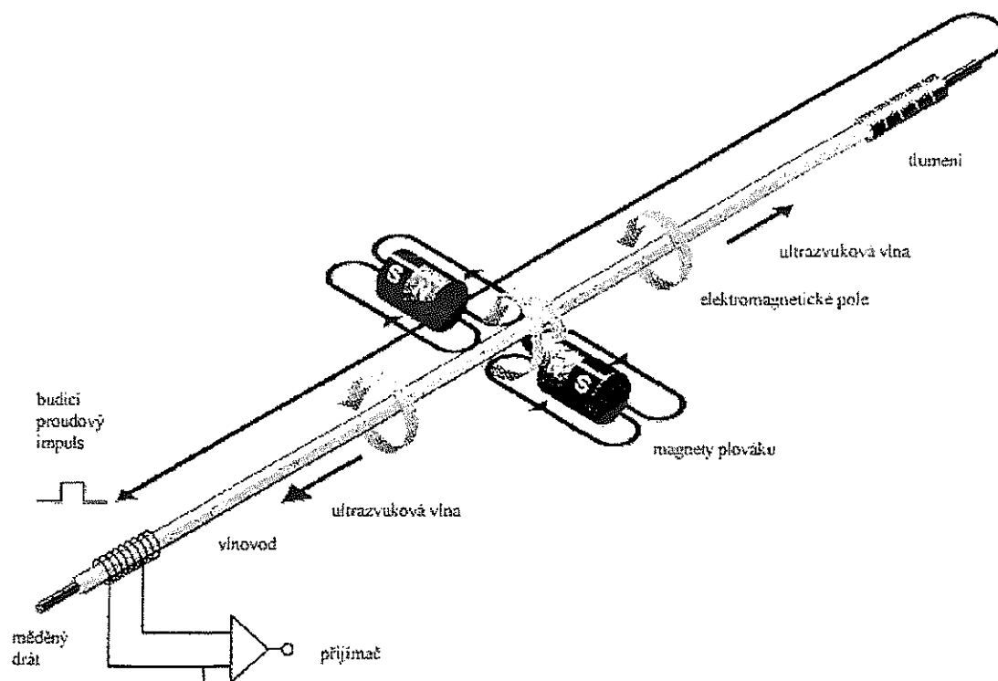
Obr.1 Princíp merania hladinomera
