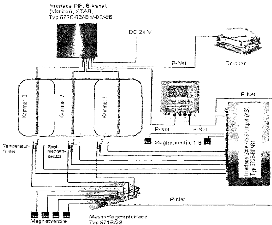
Obr. 4c Merací systém s prepočítavačom Systém (PETRODAT) 3003 s rozhraním hladinomerov
