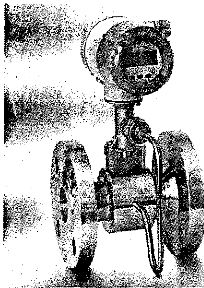
Obr.č.2 OPTISWIRL 4070 C /prírubové vyhotovenie s integrovaným snímačom tlaku/
