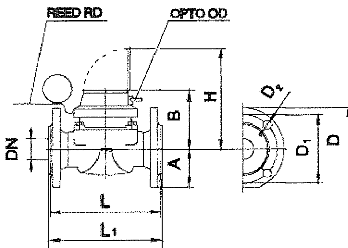
Obr.č.2 Teleso vodomera typu WP - Dynamic
