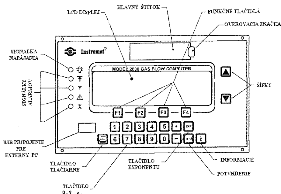
Obr. č.3 Pohľad na predný panel počítača Elster Instromet FC 2000
