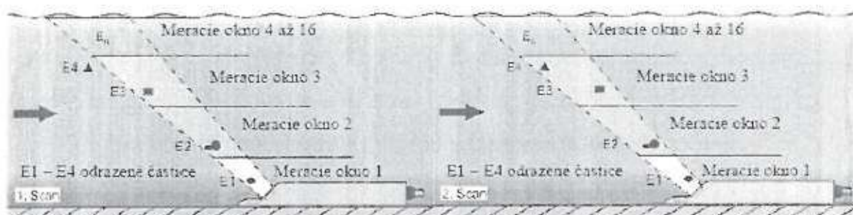
Obr. č. 4 Princíp merania rýchlosti – situácia pri prvom a druhom prijatí odrazeného signálu
