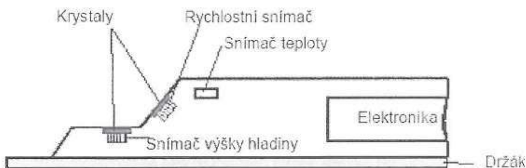
Obr. č. 3 Konštrukcia kombinovaného snímača POA-V1H1KT
