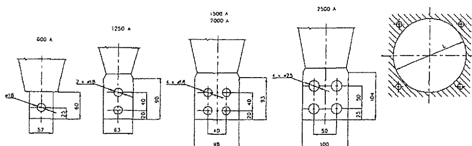
Připojovací rozměry koncových svorek
