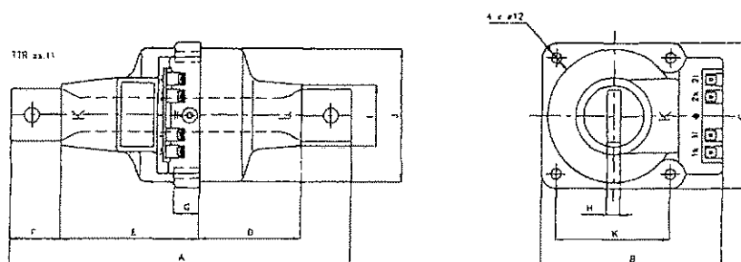
Připojovací rozměry koncových svorek
