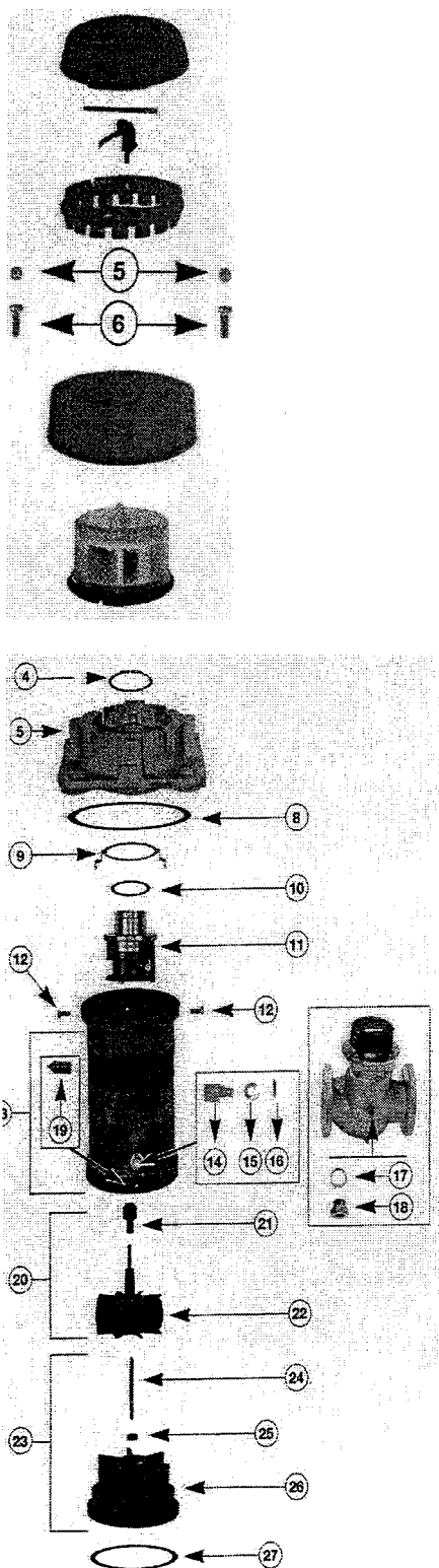
Obr.č. 4 Jednotlivé časti mechanizmu vodomera typu Voltmag V
