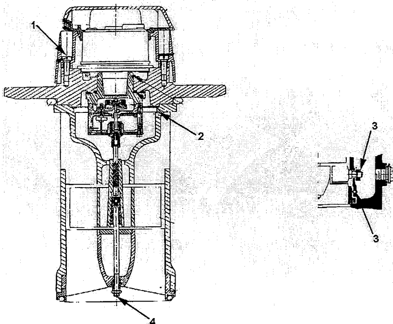
Obr.č.7 Zabezpečenie mechanizmu vodomera Woltmag V
