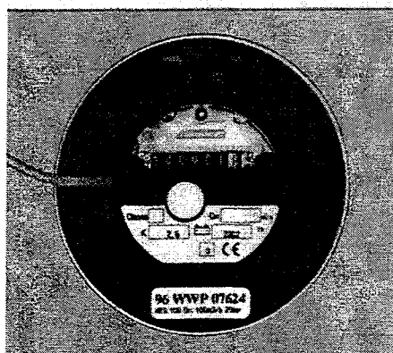
Obr. č.6 Ciferník počítadla vodomera
