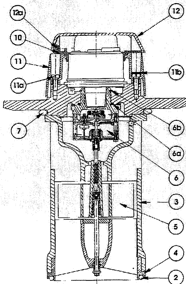
Obr.č. 5 Konštrukcia mechanizmu vodomera typu Voltmag V
