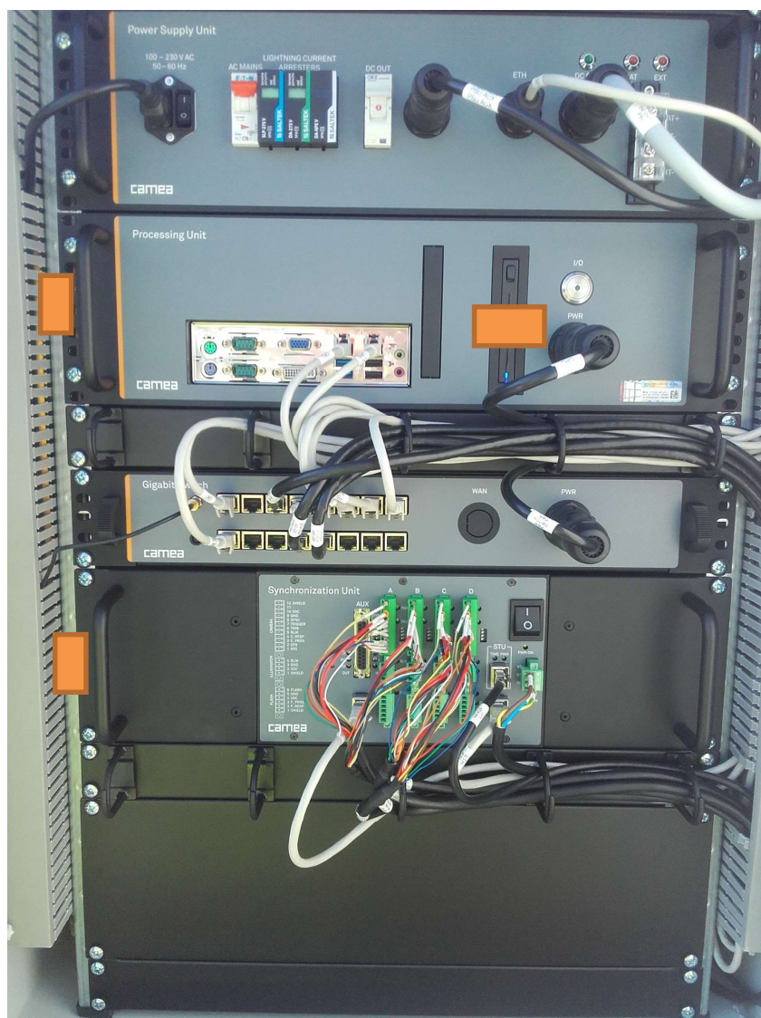
Obr. 6 Rozvodňa UC-CAB s komponentami UnicamSPEED-R (UC-PSU, UC-CPU, UC-ESU, UC-SIU, UC-SU), oranžové obdĺžniky sú vyznačené miesta pre overovacie značky
