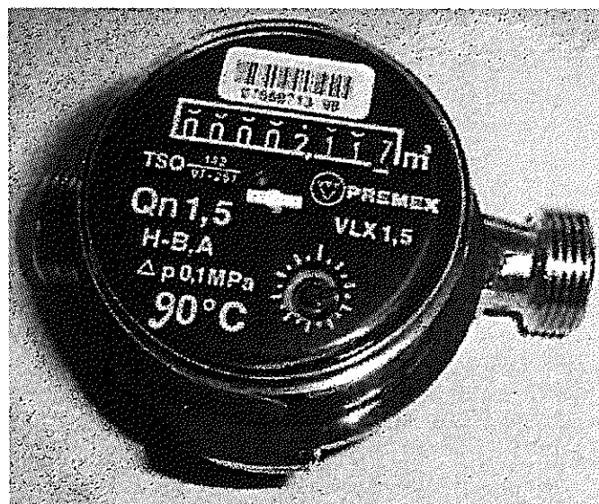
Obr. č. 1 Vodomer typu VOLUMEX VLX 1,5/90.X
