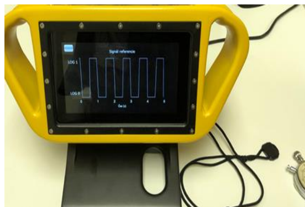
Obrázok č. 4: Zariadenie na kalibráciu stopiek priamou metódou
