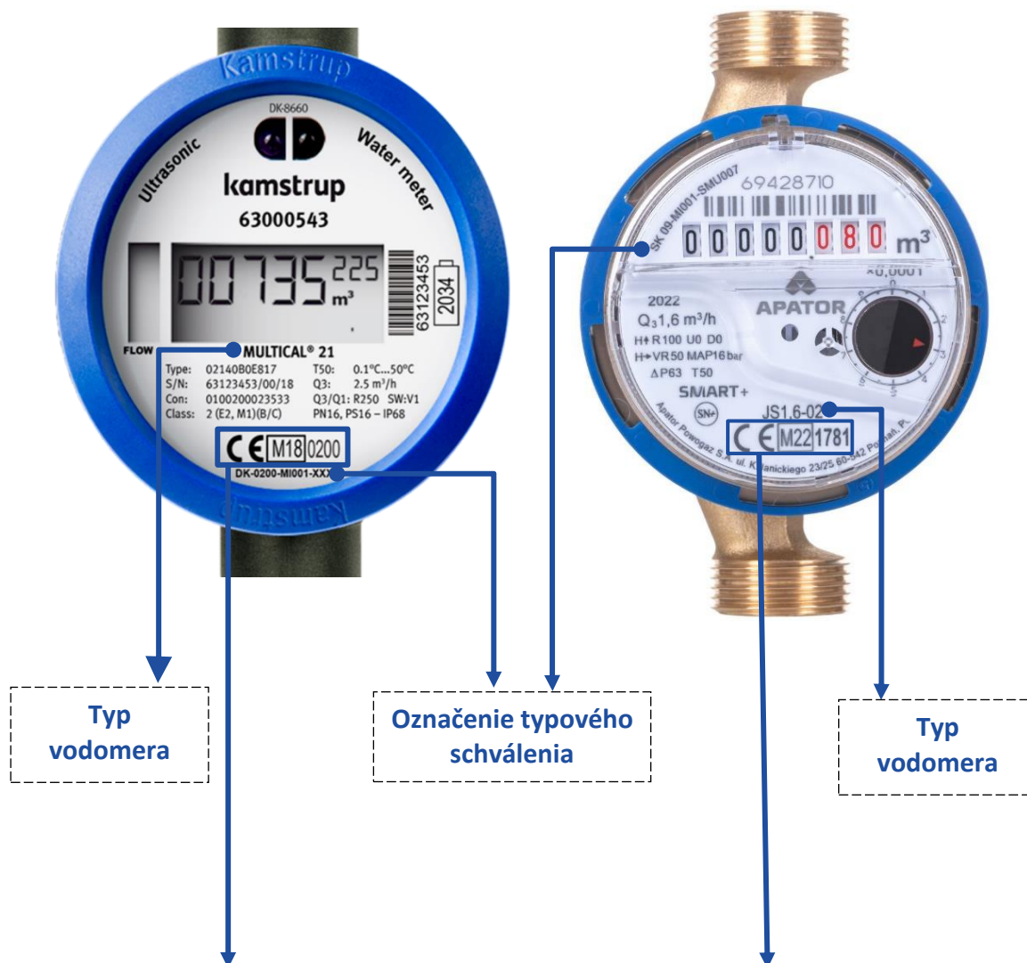
Ultrazvukový vodoměr
